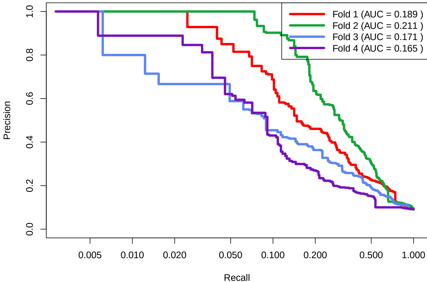
SPELL All Datasets: 430x20x1 Run 2
