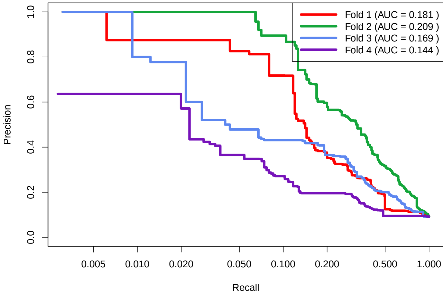
SPELL All Datasets: 430x20x1 Run 5
