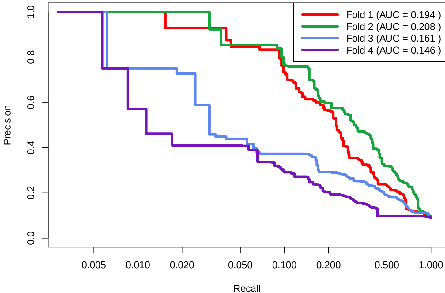
SPELL All Datasets: 430x20x1 Run 1
