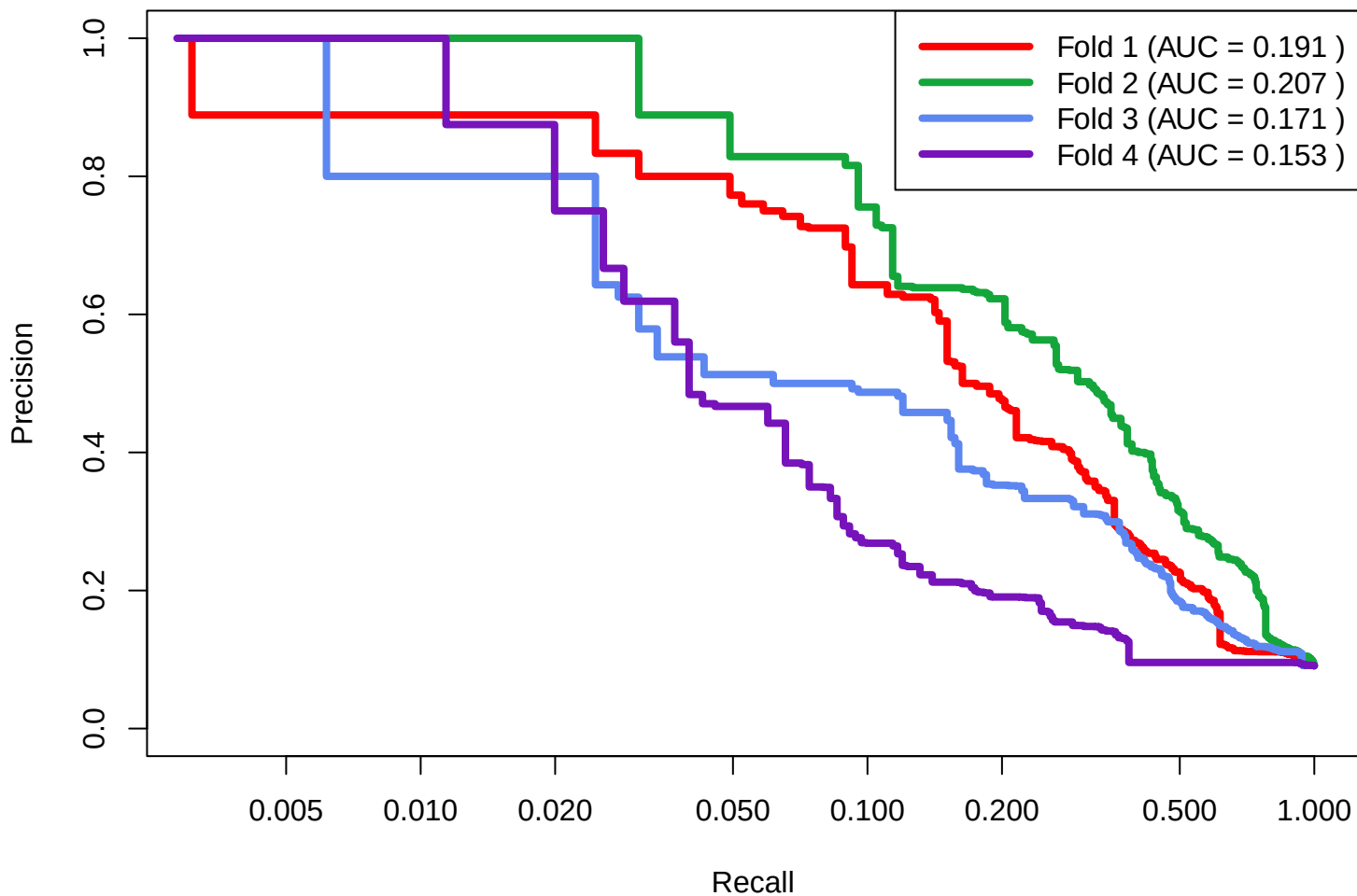
SPELL All Datasets: 430x20x1 Run 8
