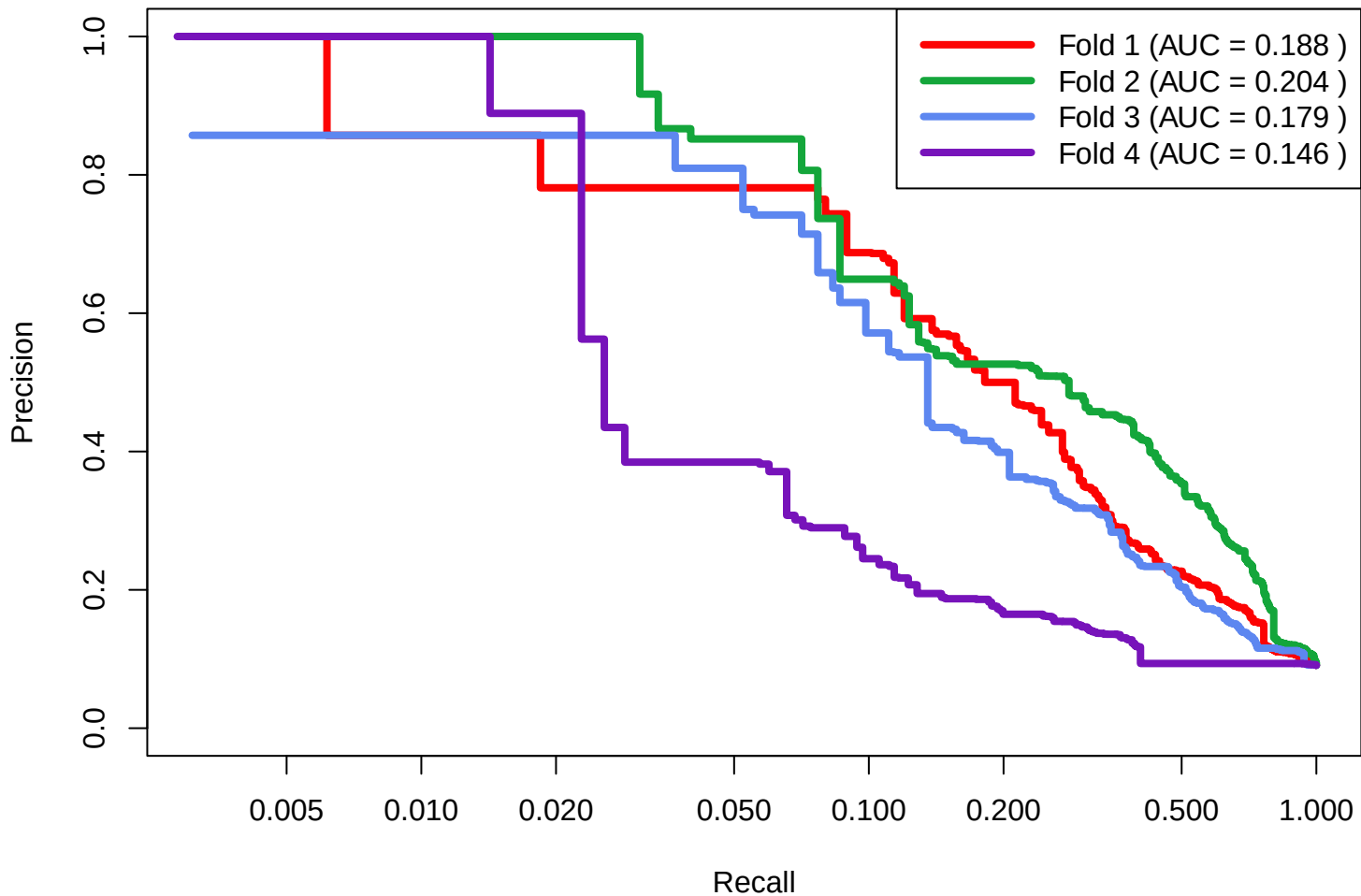
SPELL All Datasets: 430x20x1 Run 6
