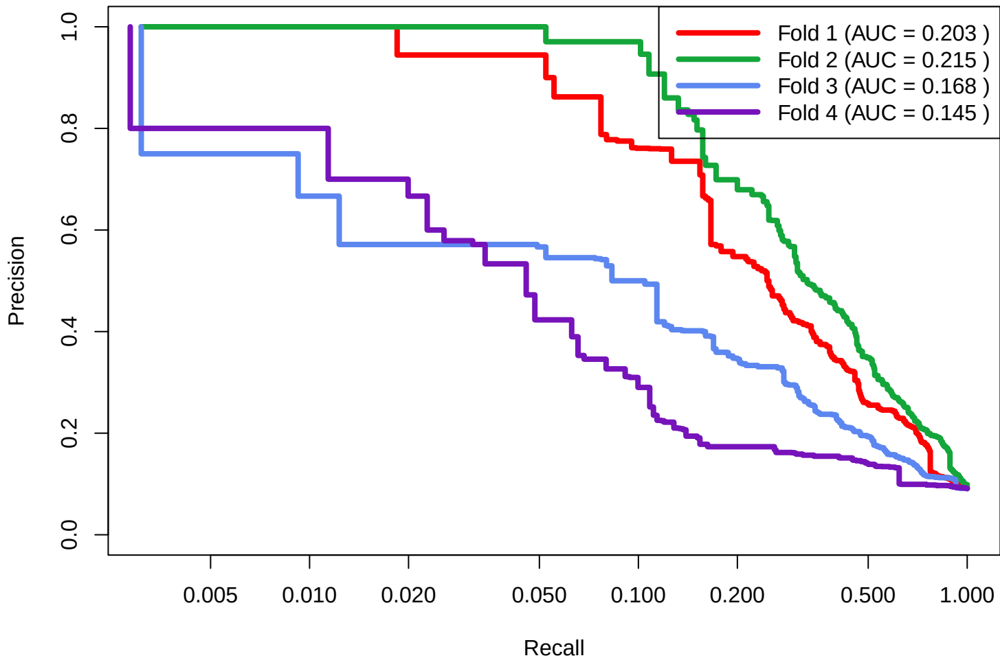
SPELL All Datasets: 430x20x1 Run 9
